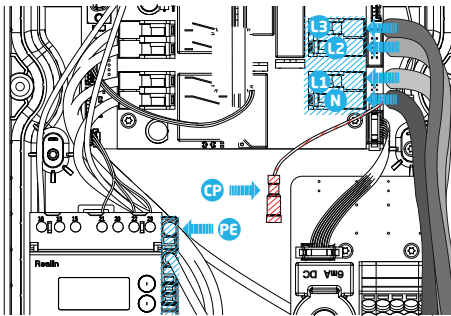
Figuur 8: Elektrische aansluiting vaste laadkabel, S-line / Pro-line, 3 fase
