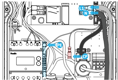
Figuur 6: Elektrische aansluiting vaste laadkabel, S-line, 1 fase
