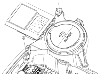
Figuur 3: Het subframe verwijderen
