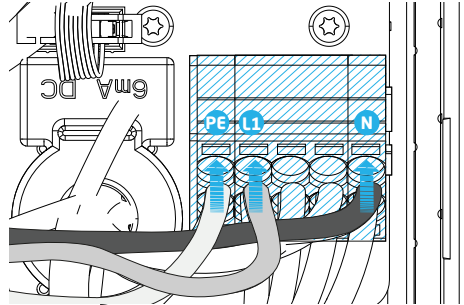
Figuur 5: Elektrische aansluiting, S-line / Pro-line, 1 fase
