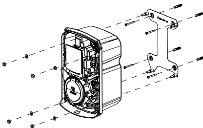
Figuur 4 Montage aan de muur
