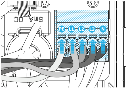
Figuur 7: Elektrische aansluiting, S-line / Pro-line, 3 fase
